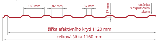
Střešní profil
