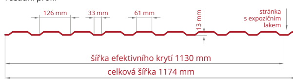
Fasádní profil
